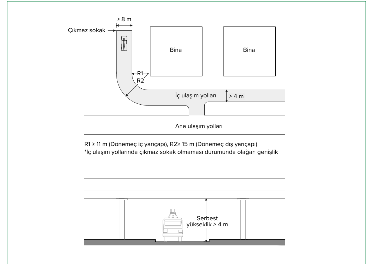
Şekil 22.3: İç ulaşım yolları
