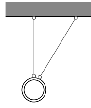
İki yollu boylamasına sabitleme askı elemanları örneği*
