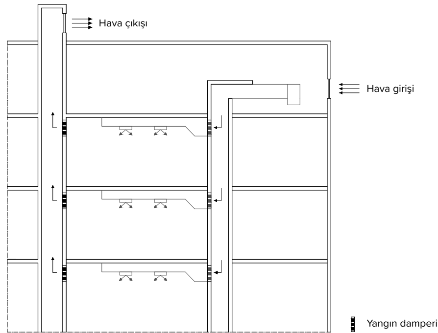
Havalandırma kanalı korunmuş bir şaft içinden geçtiği durumda şafta giriş ve çıkışta yangın damperi kullanılması
