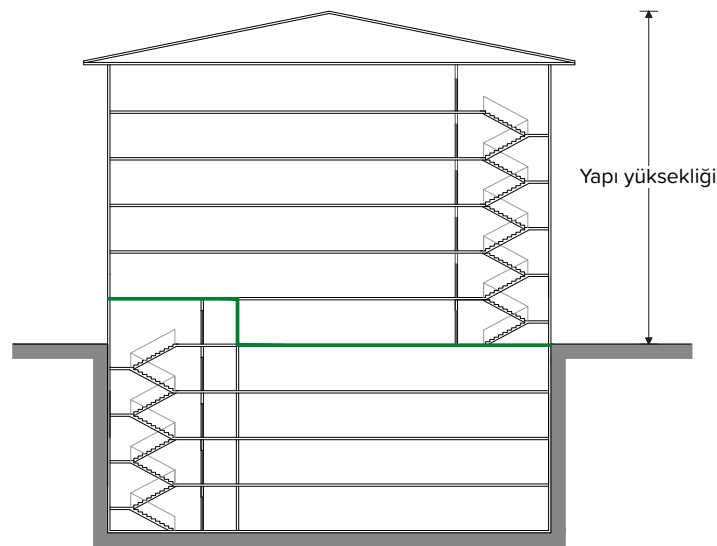
Konutlarda bodrum katların yapı yüksekliğine dahil edilmediği durum
