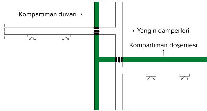
Havalandırma veya tahliye kanallarının yangın kompartıman duvarı veya katını delmesi durumunda
