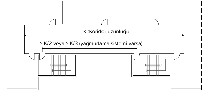
Şekil 39.4: Çıkışlar arasındaki mesafe
