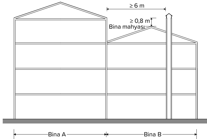
Şekil 58.2: Havalandırma bacası
