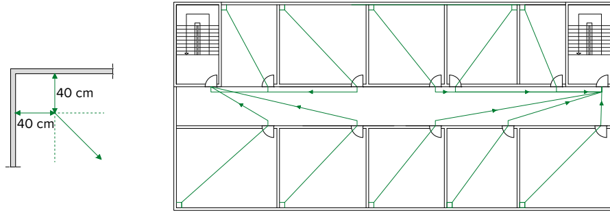
Şekil 32.6: Kaçış uzaklığı
