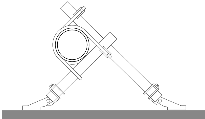
Dört yollu destek-sabitlenme askı elemanı örneği*
