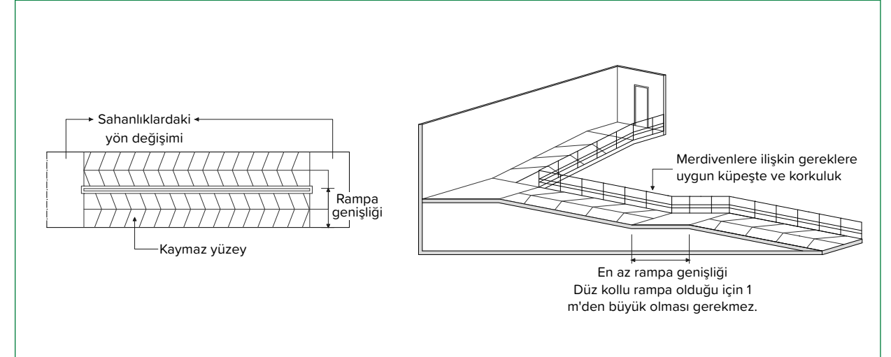
Şekil 44.1.b: Kaçış rampaları
