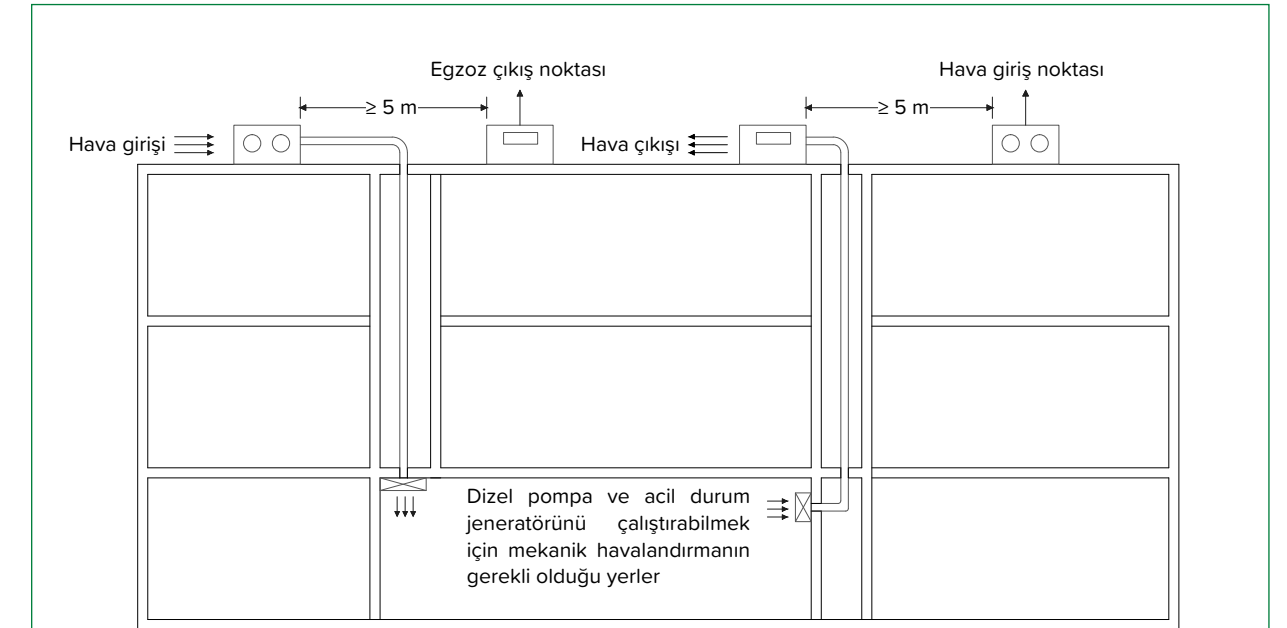
Şekil 88.1: Duman tahliye sistemleri
