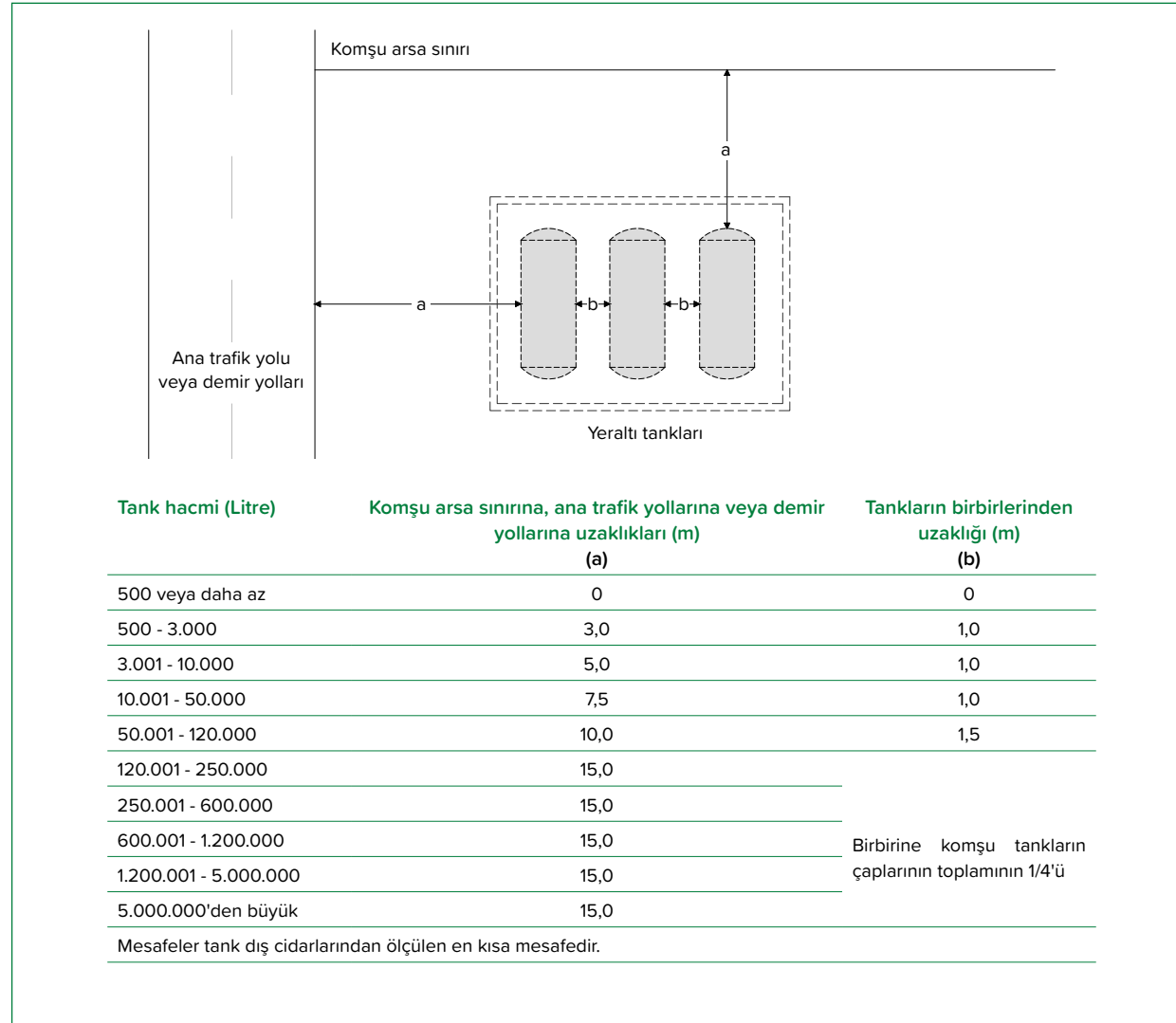
Şekil 120.2.b: Ek-12/Ç Yeraltı Tankları ile İlgili Asgari Emniyet Mesafeleri
