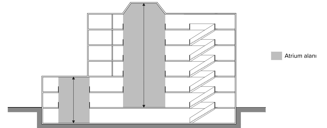
Şekil 4.g: Atrium
