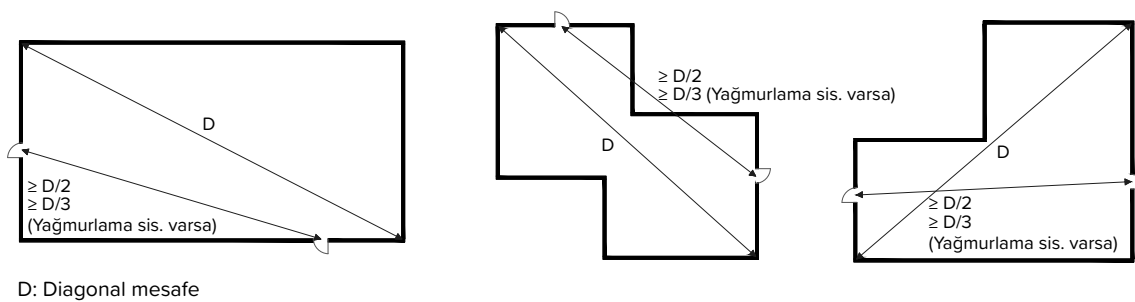
Şekil 39.3: Bölünmemiş tek mekanlarda çıkışlar arasında mesafe
