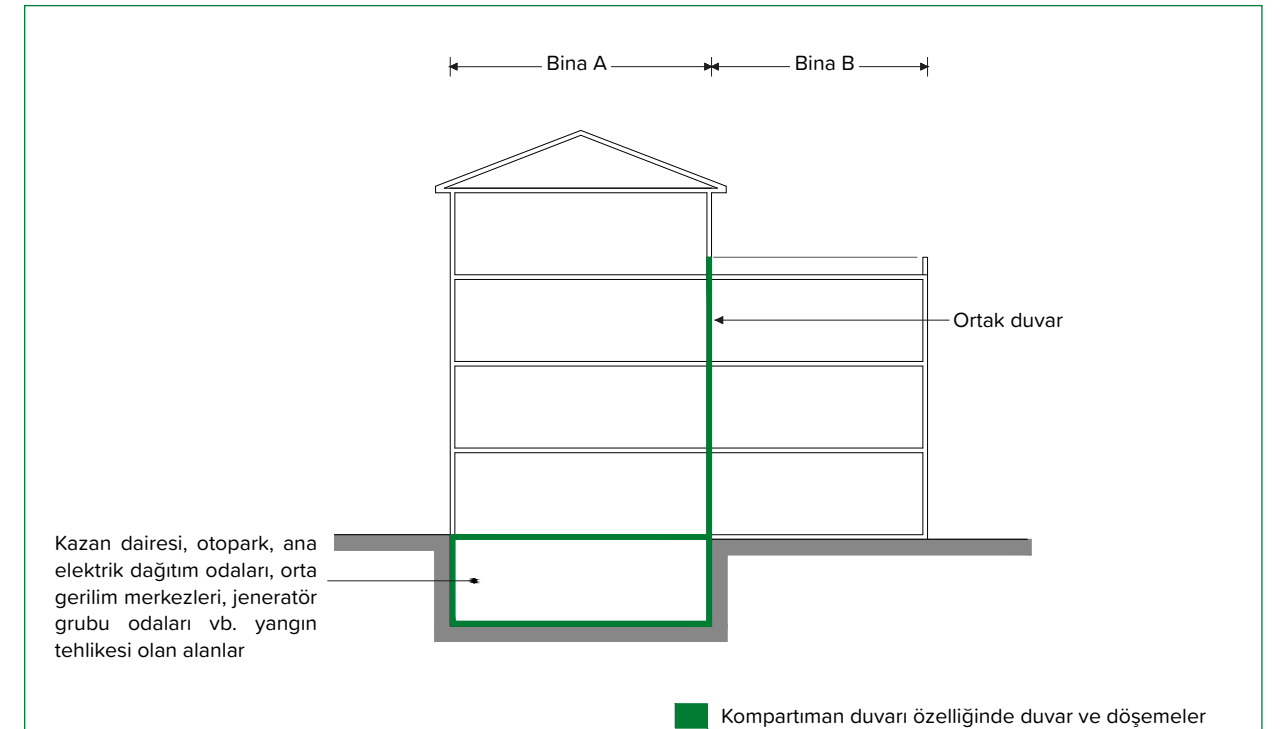
Şekil 24.2: Yangın kompartımanları
