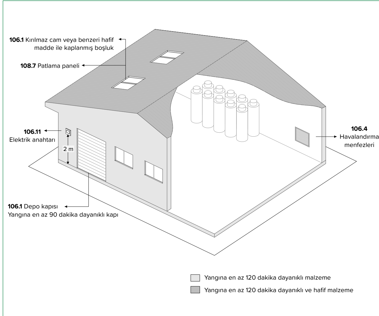
Şekil 106.1-4-11: LPG depolanacak binalar ile ilgili güvenlik önlemleri
