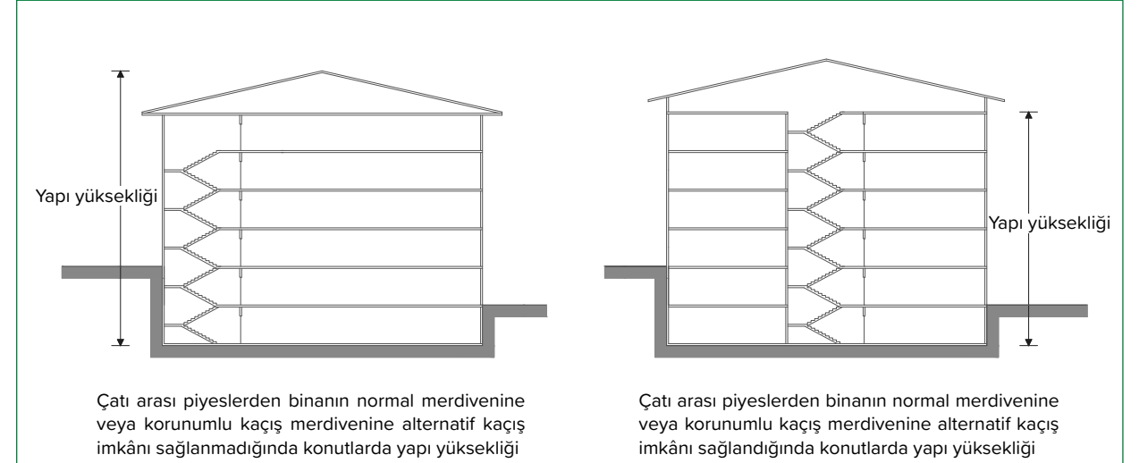
Şekil 48.8: Konutlarda yapı yüksekliği istisnası
