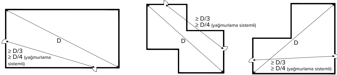
Şekil 150.1.b: Mevcut yapılarda bölünmemiş mekânlarda kapılar arasındaki mesafe
