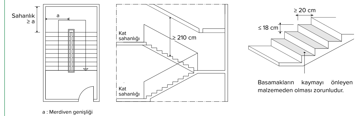
Şekil 152.1: Mevcut yapılarda kaçış merdiveninin özellikleri
