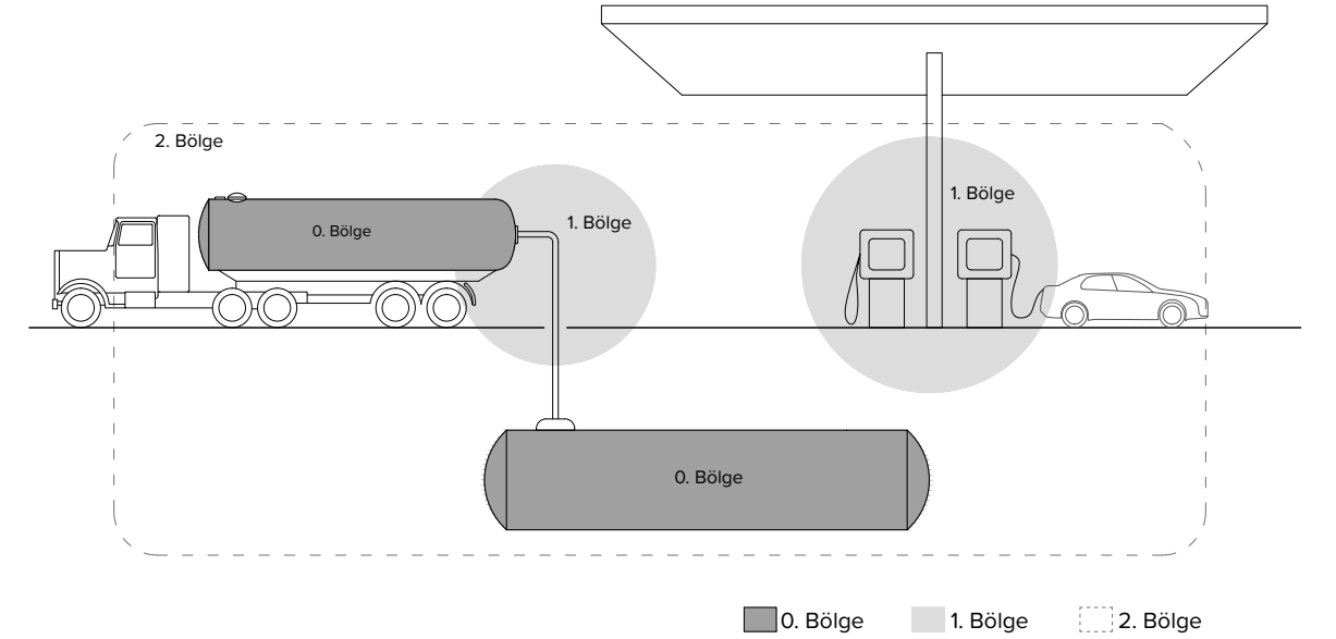
Şekil 116: Tehlike Bölgeleri
