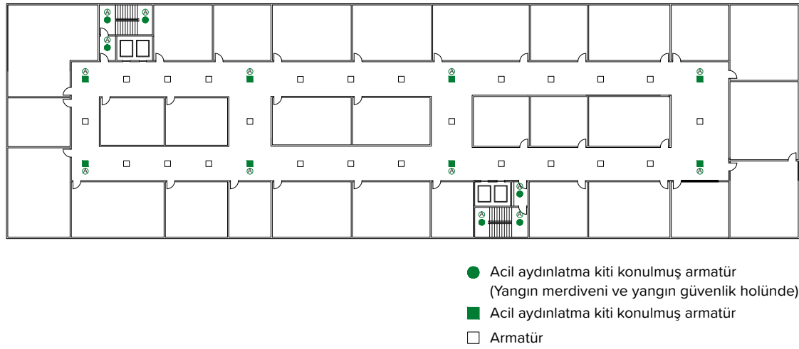
Şekil 71.2: Kaçış yollarının aydınlatılması
