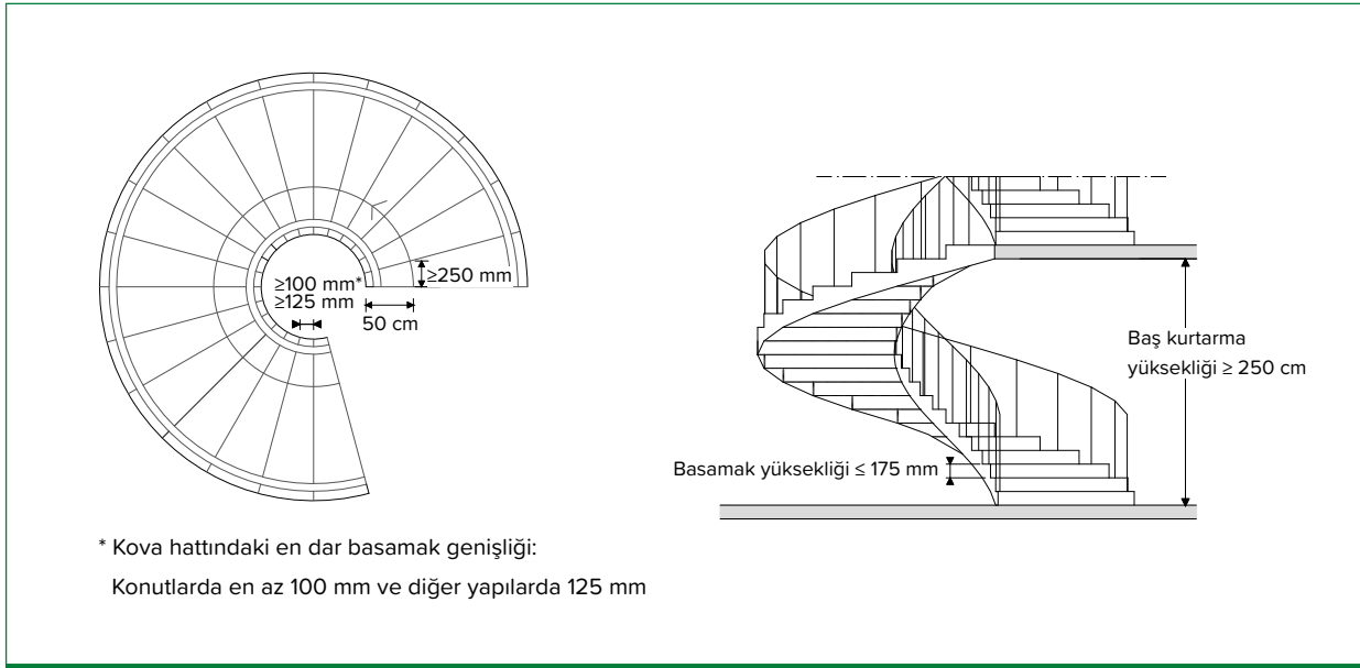
Şekil 43.2-3-4-5: Dairesel merdiven
